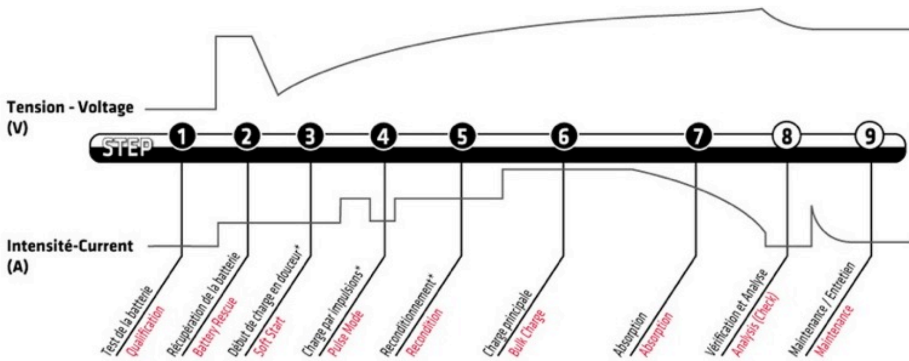
Les phases 2, 3, 4 et 5 sont les phases de désulfatation Steps 2, 3, 4 and 5 are desulfation steps
